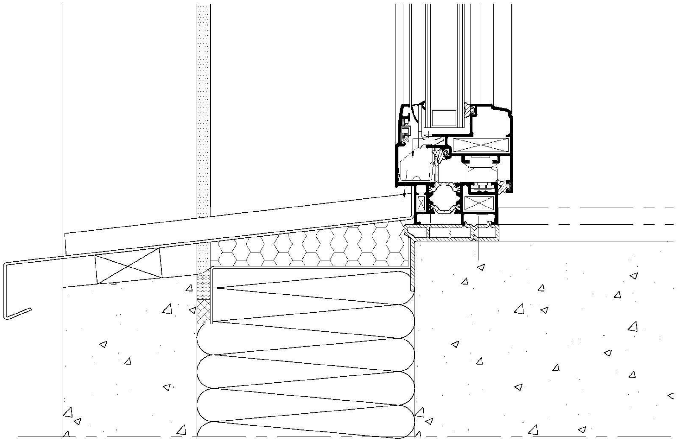
Jonction menuiserie-panneau coupe verticale appui
